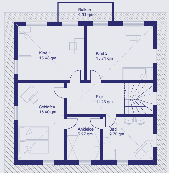
Dachgeschoss
